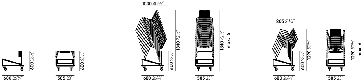
HAL Stapelwagen, Für alle stapelbaren HAL geeignet (ausser HAL A-Stacker)
